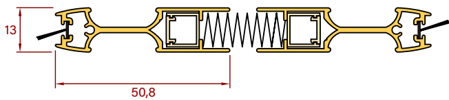
Griffschiene
