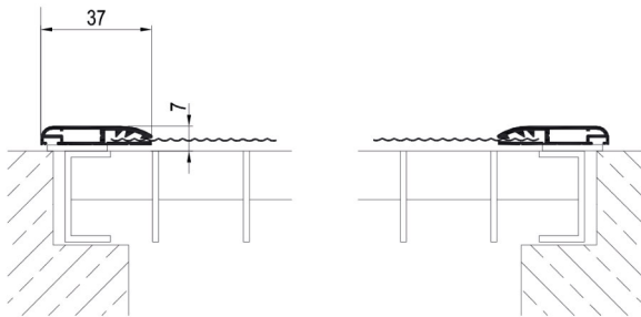
Schnitt bei Montage ohne Wandanschlussbürste
