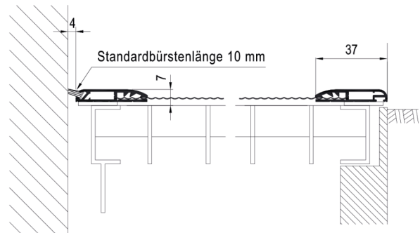
Schnitt bei Montage mit Wandanschlussbürste
