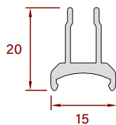
Führungsprofil
